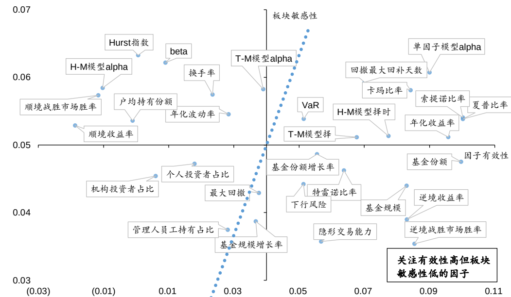
图表27：选基因子的有效性和板块敏感性
